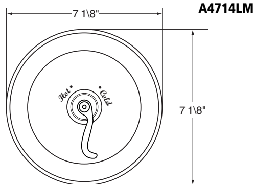
A4714LM
