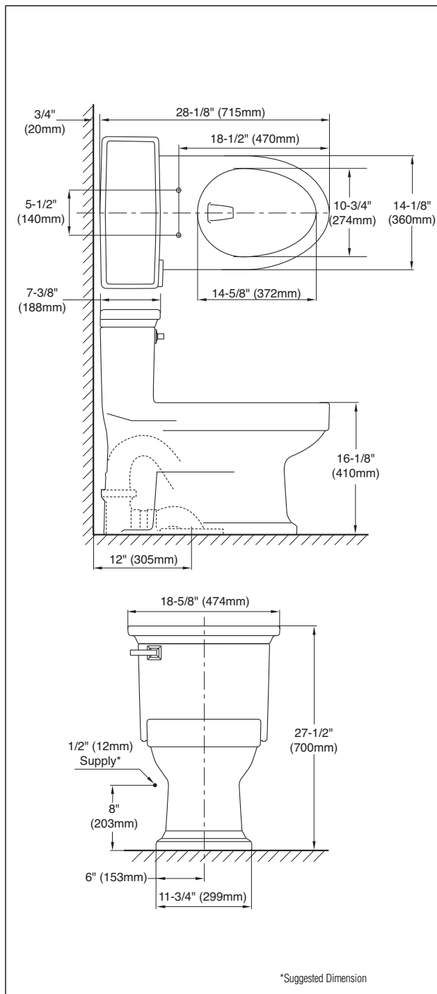
MS934214SF - Lloyd™ Toilet
